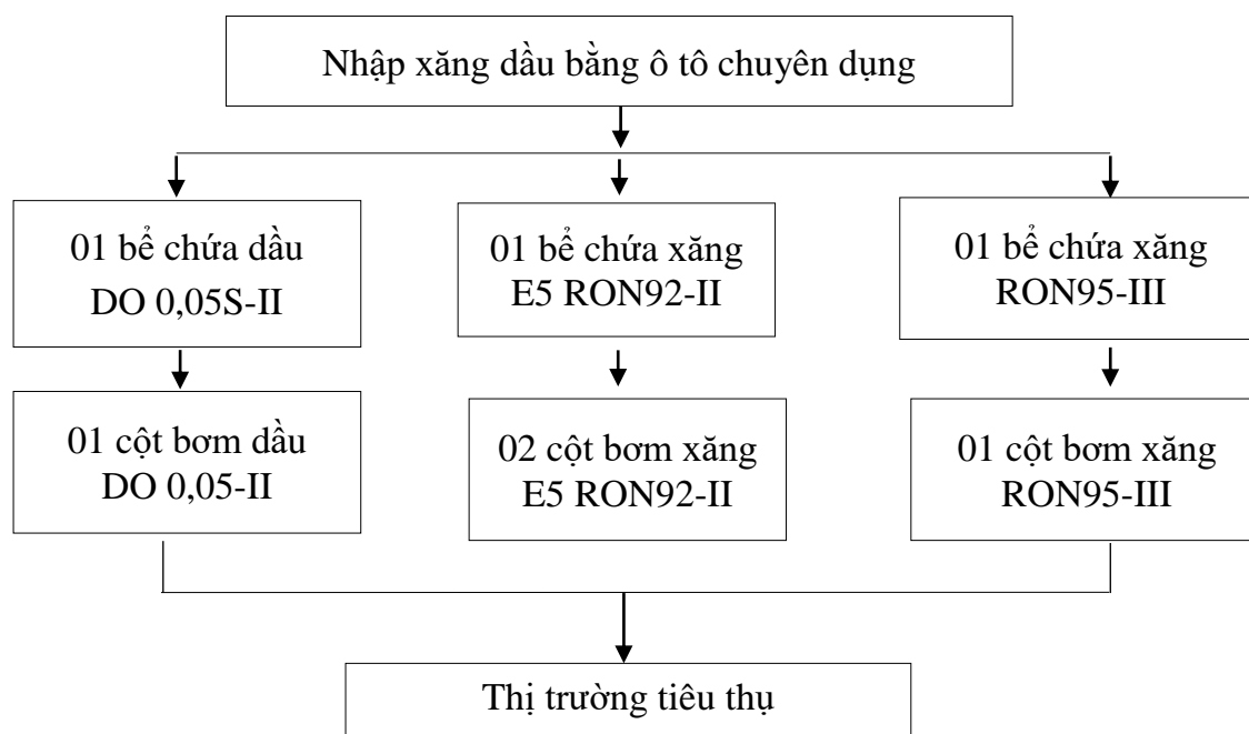
Sơ đồ 1.1. Quy trình công nghệ xuất nhập xăng dầu của Cơ sở
