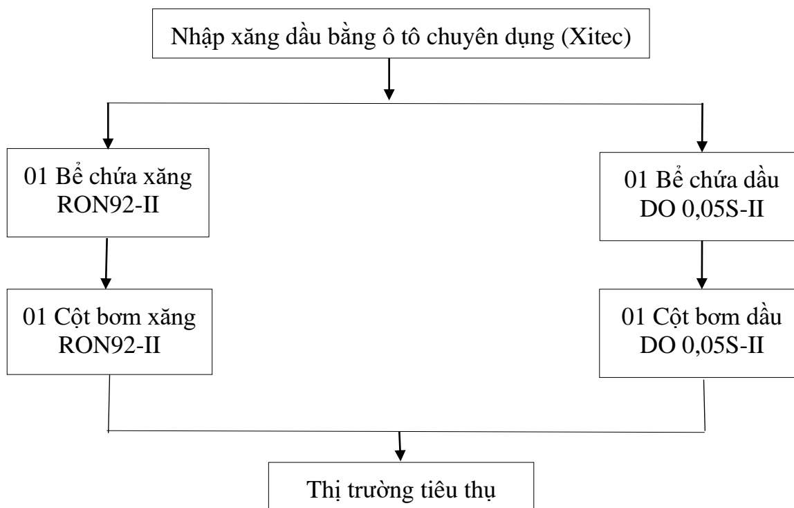
Hình 1.1. Sơ đồ quy trình công nghệ xuất nhập xăng dầu của Cơ sở
